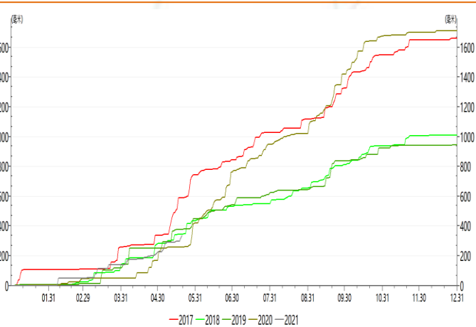
图 8：泰国:东部:罗勇:累计降雨量
