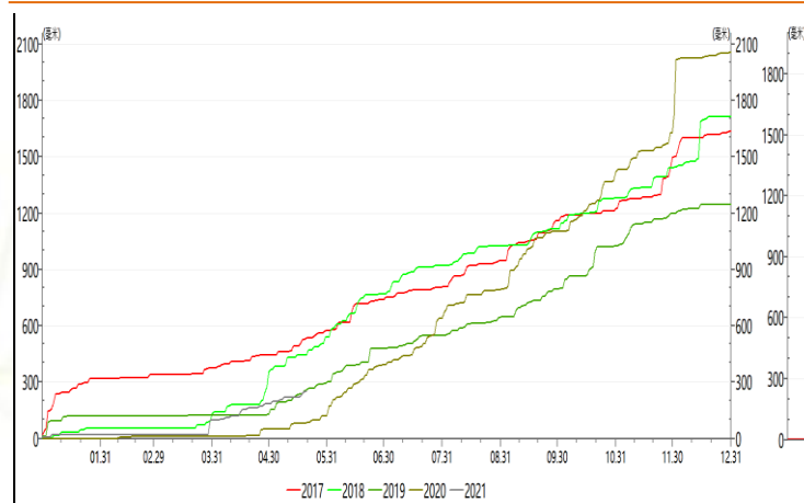
图 5：泰国南部(东海岸):叻他尼府:累计降雨量
