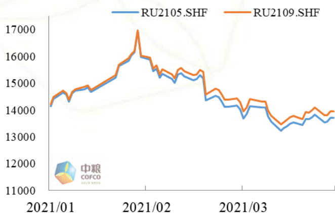
图 1: 沪胶 2105 及 2109
