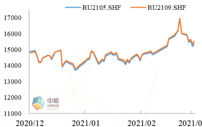
图 1: 沪胶 2105 及 2109
