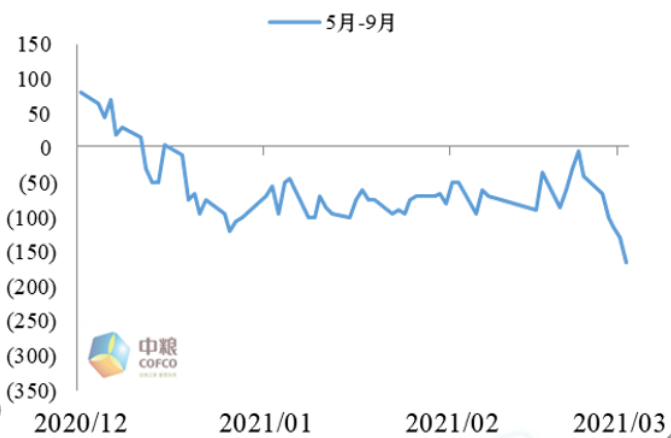
图 2: 沪胶 5 月-9 月
