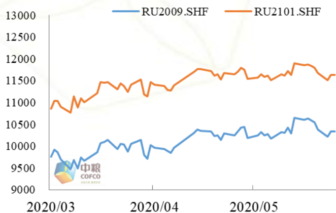
图 1: 沪胶 2009 及 2101
