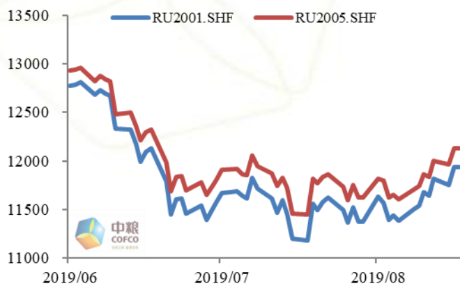
图 1: 沪胶 2001 及 2005
