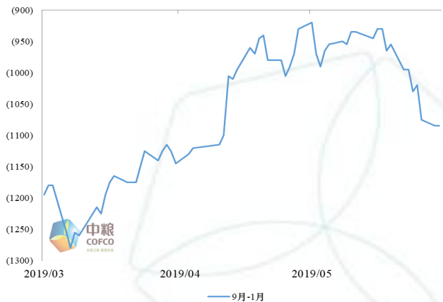
图 2: 沪胶 9 月-1 月
