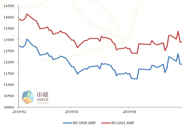
图 1: 沪胶 1909 及 2001
