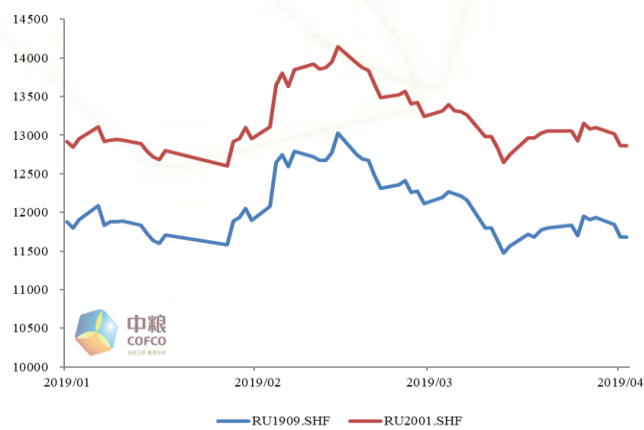
图 1：沪胶 1909 及 2001
