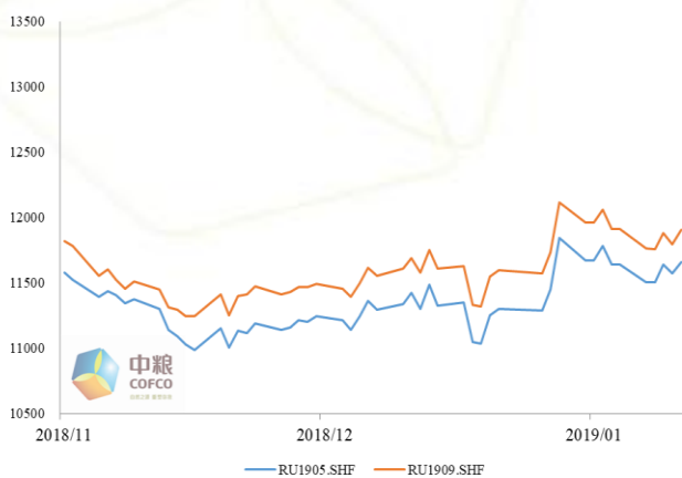
图 1: 沪胶 1905 及 1909
